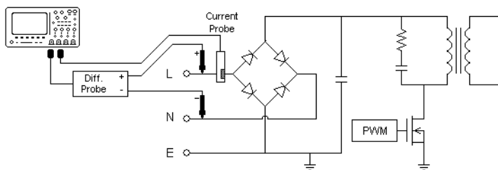
図 6 入力ライン解析テストの代表的な構成
