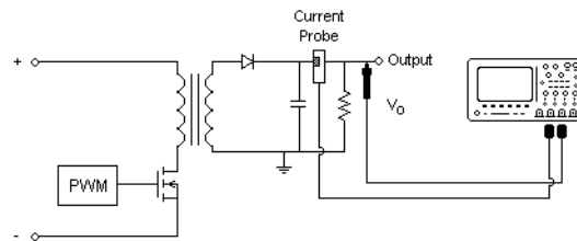
図 9 パワー出力過渡応答の代表的な構成
